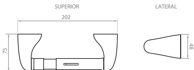
Portarrollo:
