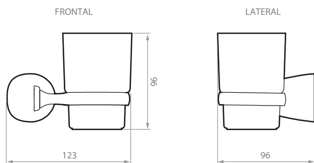
Cepillera vaso:
